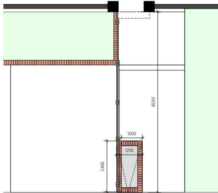
PLAN 1:50
