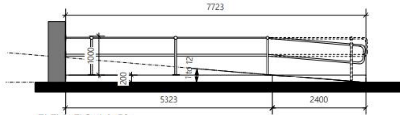
ELEVATION 1:50
