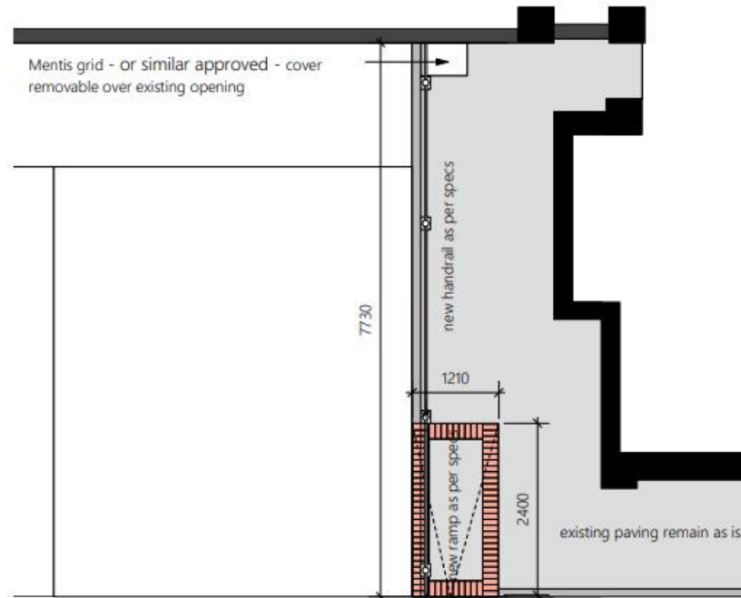
PLAN 1:50
