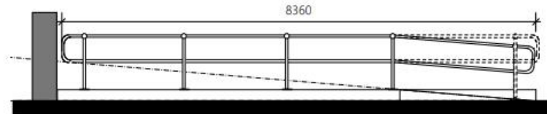
ELEVATION 1:50
