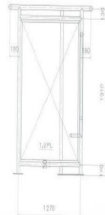
RIGHT ELEV
