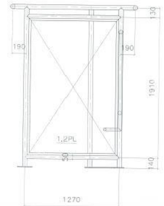
RIGHT ELEV
