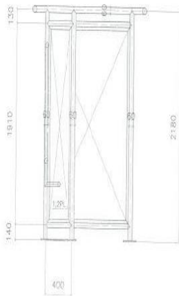
LEFT ELEV
